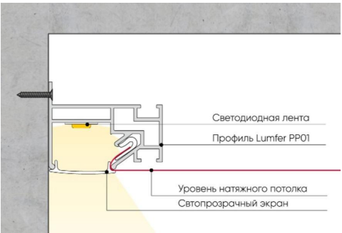
Рис.1 "Крепление светодиодных линий"
