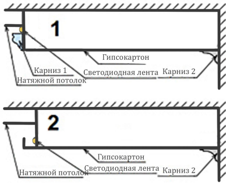
Рис.2 "Крепление светодиодной ленты в короб ГКЛ"
